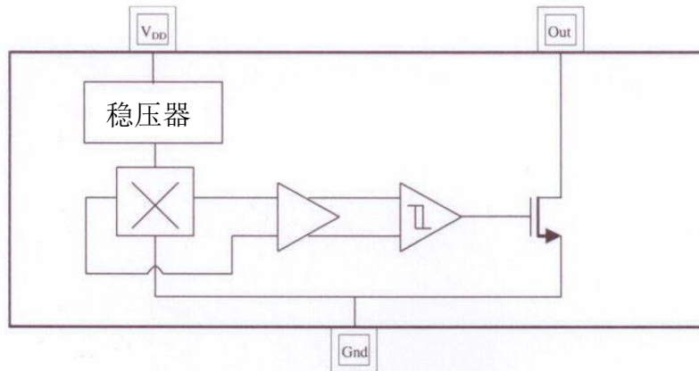
图 1 功能框图
