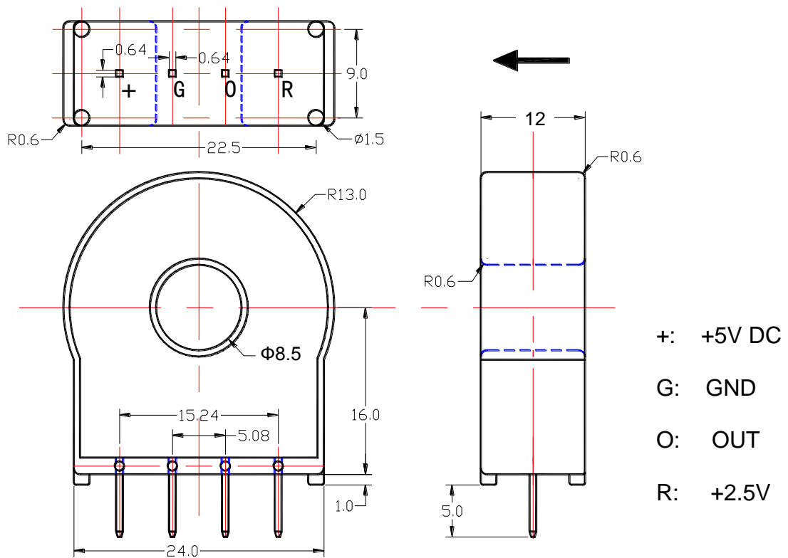
Fig. 3 Dimensions of CYHCS-ES5A
